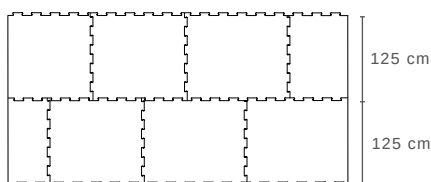
Puzzelranden aan 3 / 4 zijden
